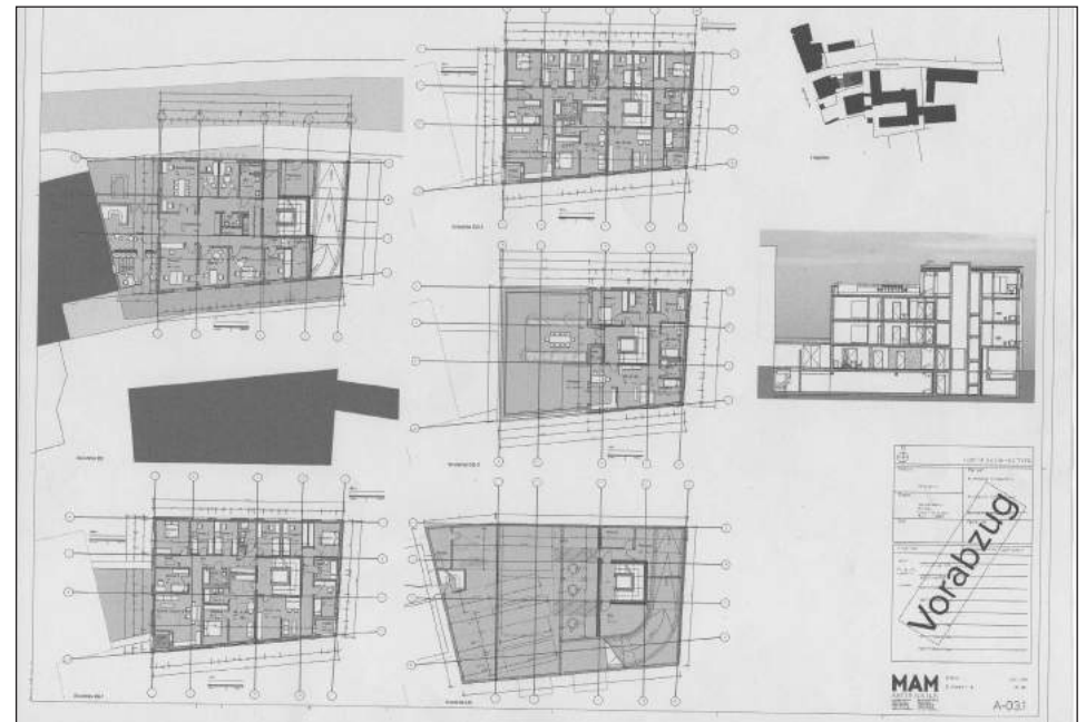
Pläne vom Pfarramt, den Wohnungen in den Obergeschossen und Tiefgarage (Plan: MAM)
