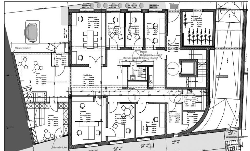
Grundriss des künftigen Pfarramtes. Links: Eingangsbereich mit Foyer + Sakristei. Oben: Besprechungsraum, Büros für Flüchtlingsintegrationsberatung, Jugendreferentin, Kantoren. Mitte: Toilette, Wartebereich, Teeküche. Unten: Pfarramt mit Theke, Büro 1. Pfarrstelle, Büro 2. + 3. Pfarrstelle, Registratur, Toilette + Putzraum.
